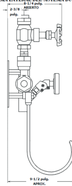
ESQUEMA LATERAL DEL SISTEMA DURAMIX
