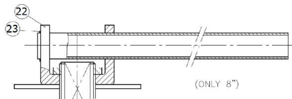
Detalle de la maneta de 8".
